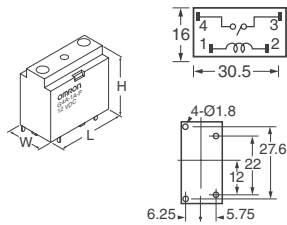
Fig. 20 - G4A
