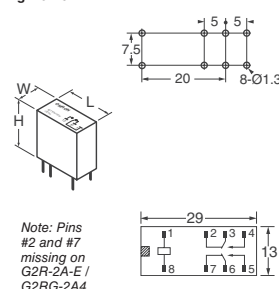
Fig. 17 - G2R-1A-E
