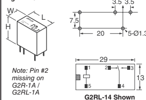
Fig. 14 - G2R-1
