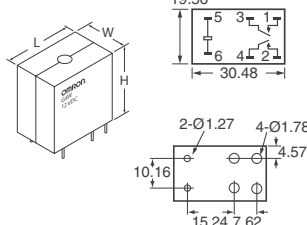
Fig. 22 - G4W
