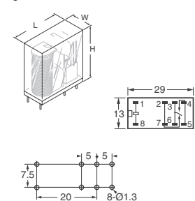
Fig. 18 - G5RL
