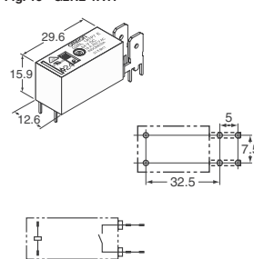
Fig. 15 - G2RL-1ATP
