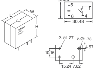
Fig. 21 - G4W
