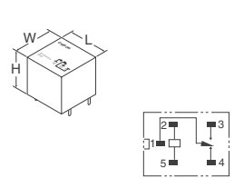
Fig. 23 - G5LA / G5LB / G5LE
