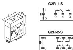
Fig. 12 - G2R-S
