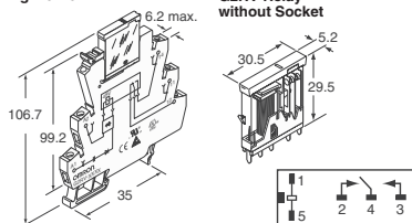
Fig. 13 - G2RV
